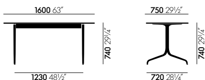
Tisch rechteckig, 1600 x 750 mm
